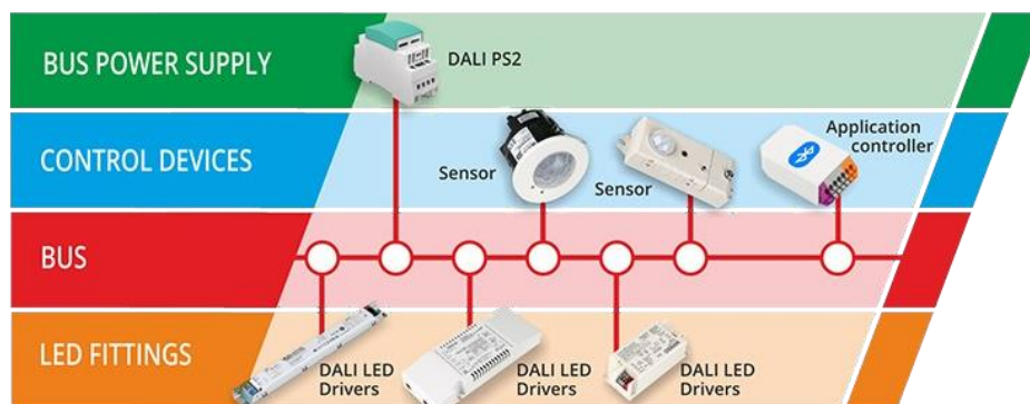
Slika 5 Inteligentni sustav upravljanja korištenjem DALI sustava iv
